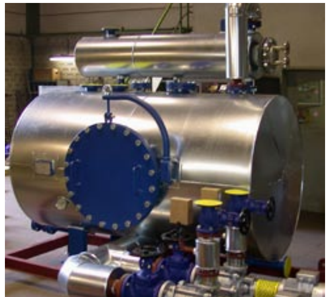
Kondensat-sammel und Rückspeiseanlage Typ SDL
