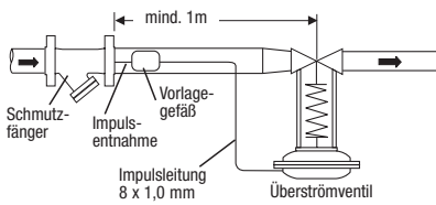
Einbauschema
