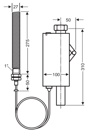
Sicherheitstemperaturbegrenzer SH4S
